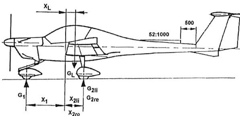
Skizze für Schwerpunktwägung
