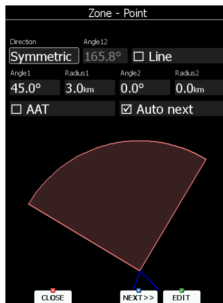
Beispiel eines FAI-Fotosektors am Wendepunkt
