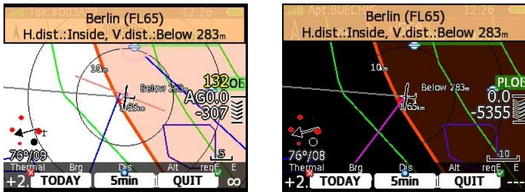
Beispiele von Luftraumwarnungen niedriger Stufe in der Clubversion auf einfarbigem Hintergrund
